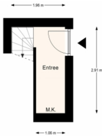
Morelstraat 24, Den Haag | 1e Verdieping H = 2.94 m
